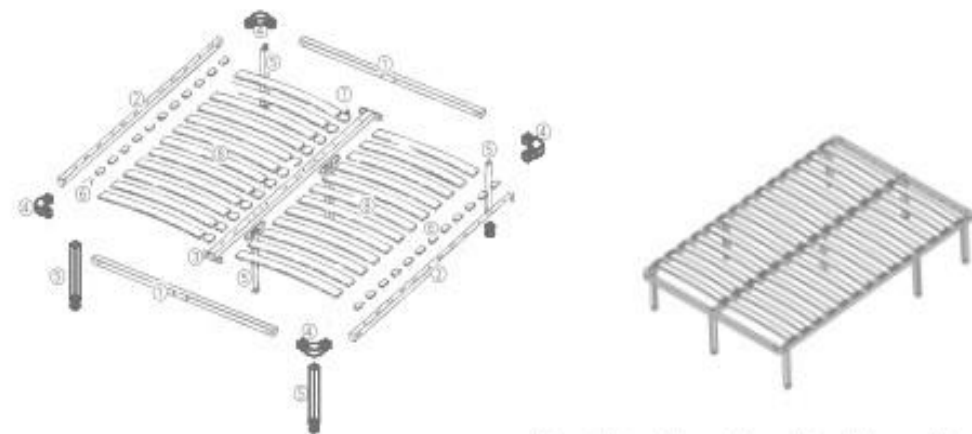
可拆分排骨架爆炸图
