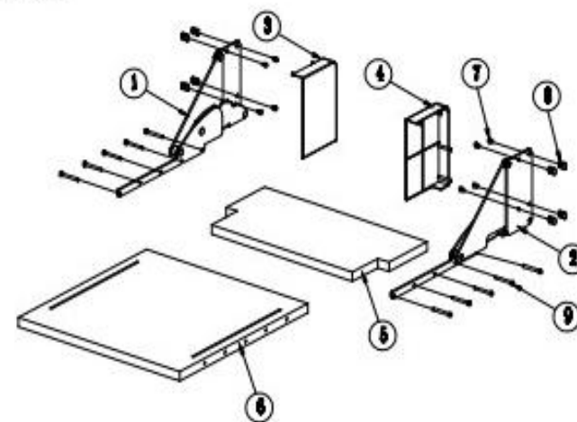
下翻面板爆炸图
